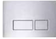
Plaza dual flush push plate 210(w) x 138(h) x 85(d)mm
